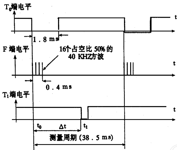
图1 测量原理时序图
