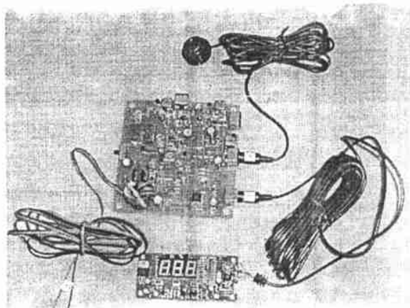
图5 汽车倒车测距仪的实物照片
