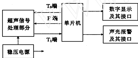
图2 系统框图
