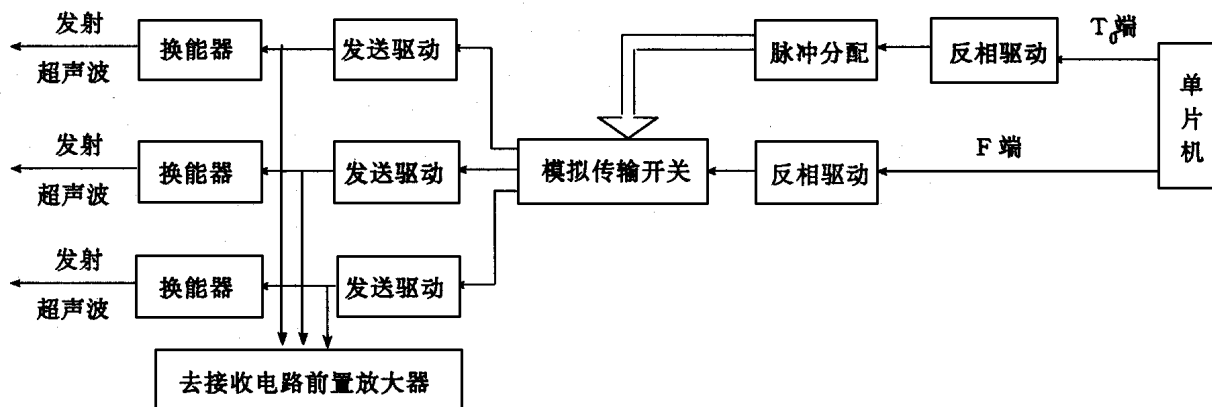
图3 超声脉冲发射电路框图
