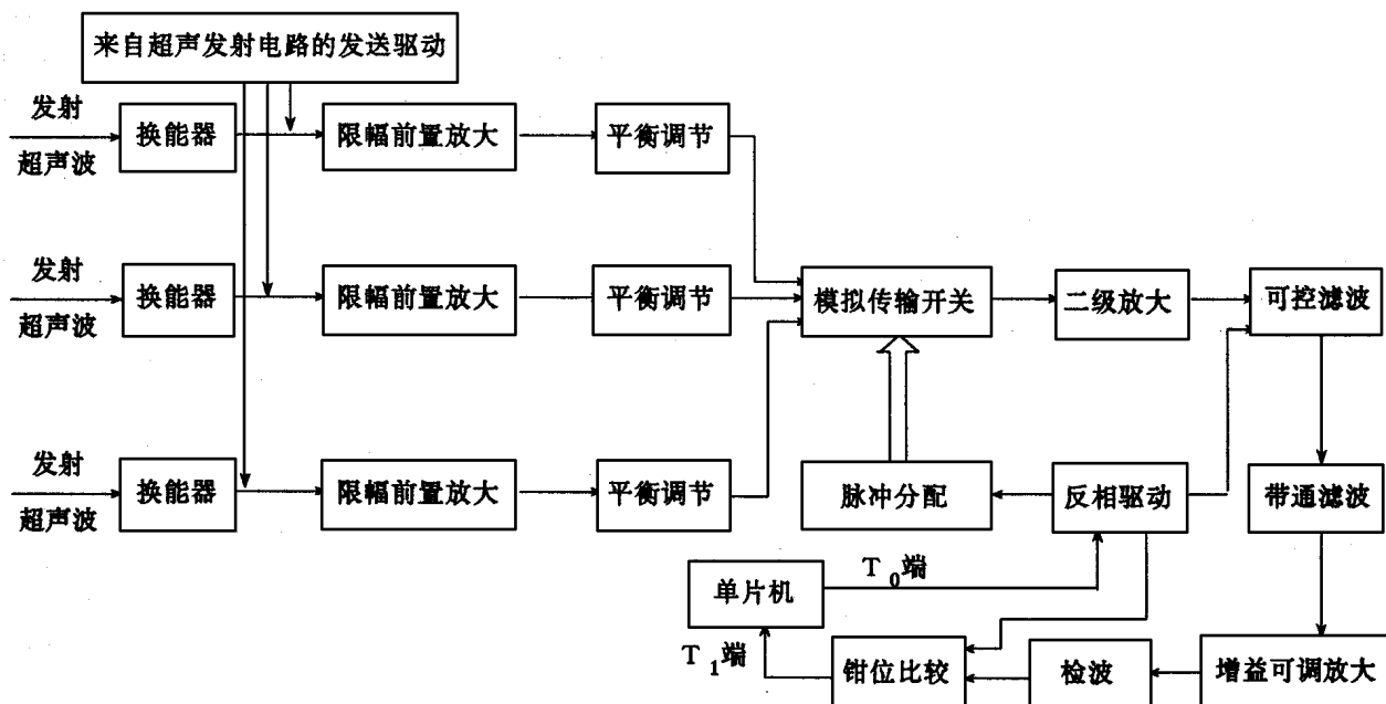
图4 超声回波接收电路框图
